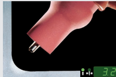
Tungsten uç çapı: 3,2 mm Temel işlem maddesi: AlMg3 Malzeme kalınlığı: 5 mm Kaynak akımı: 185 A Kaynak gerilimi: 15,6 V AC Balans: 0
